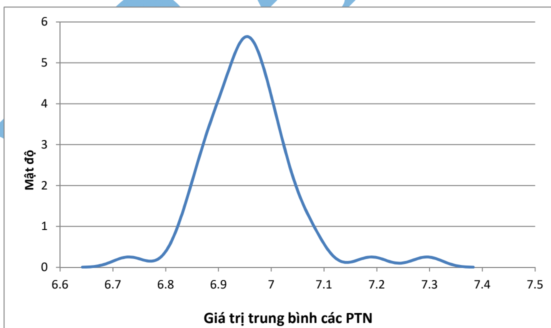
Hình 2. Biểu đồ Kernel density của mẫu B
