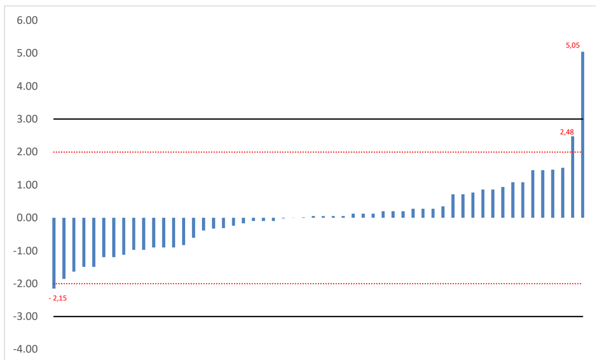
Hình 3. Biểu đồ Bar-plots của mẫu A
