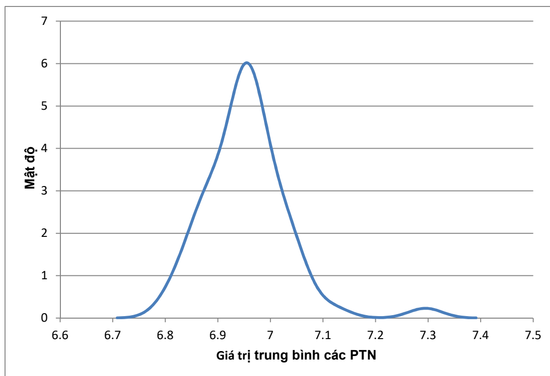
Hình 1. Biểu đồ Kernel density của mẫu A
