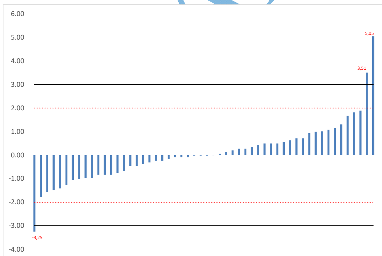
Hình 3. Biểu đồ Bar-plots của mẫu A
