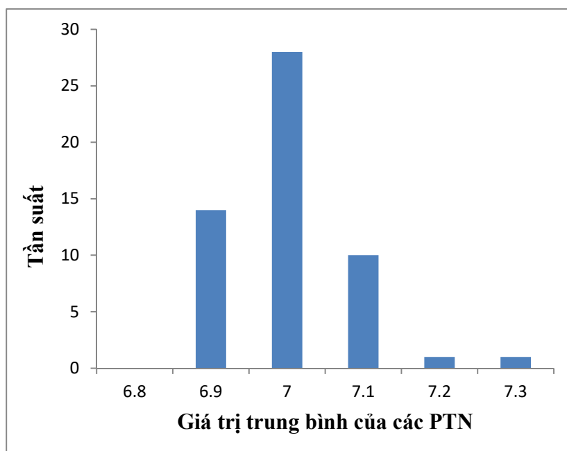
Hình 1. Biểu đồ Histogram của mẫu A
