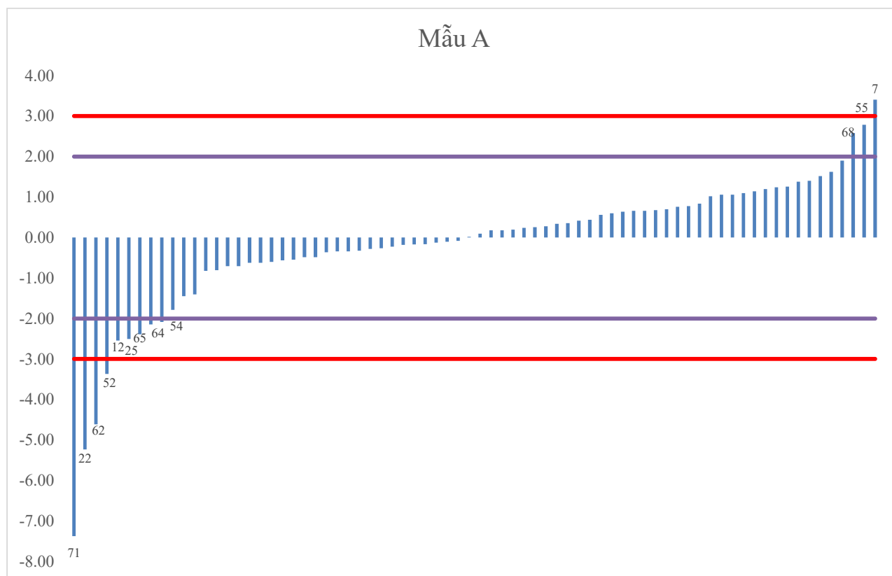
Hình 5. Biểu đồ Bar-plots của mẫu A
