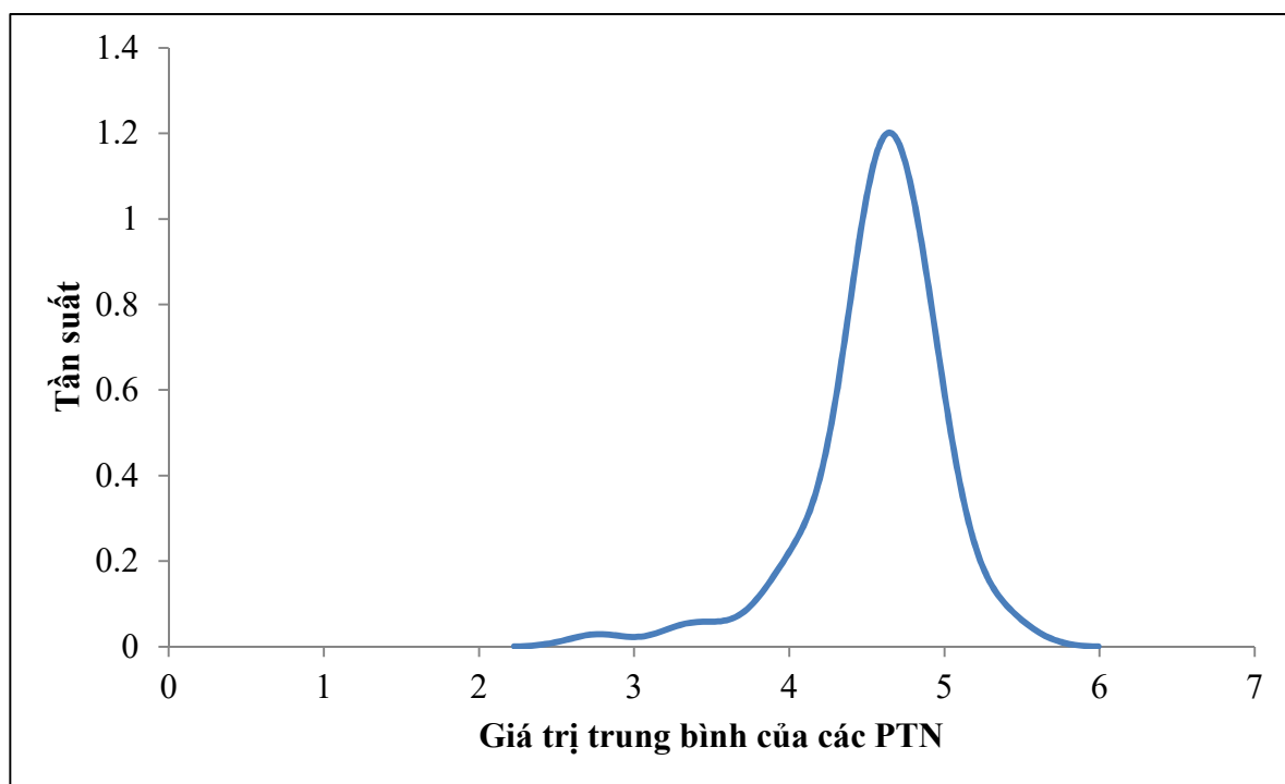
Hình 3. Biểu đồ Kernel của mẫu A
