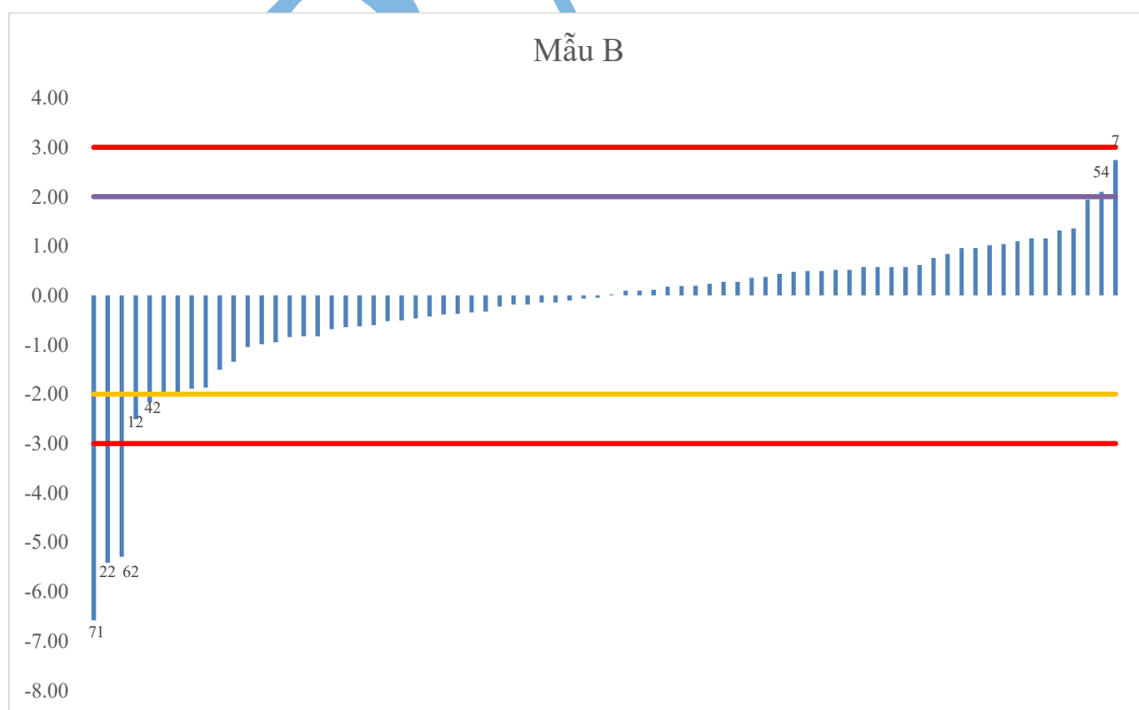
Hình 6. Biểu đồ Bar-plots của mẫu B
