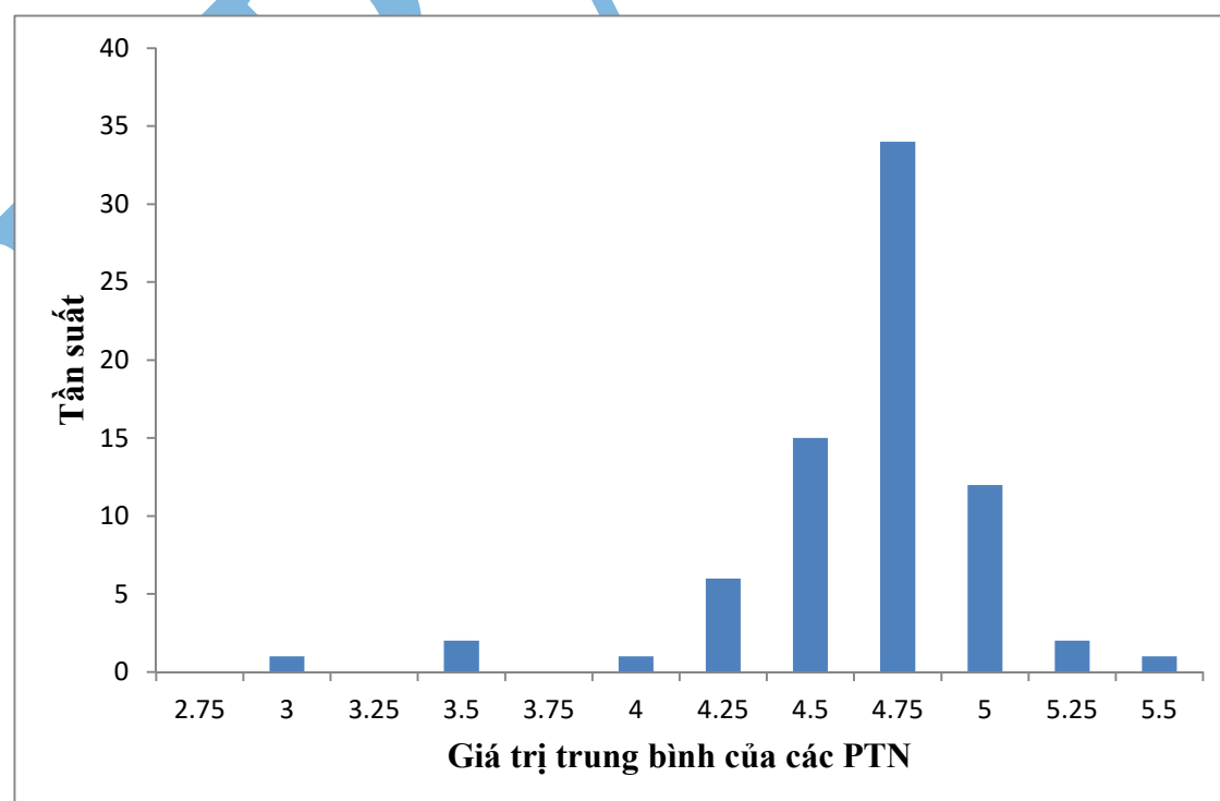
Hình 2. Biểu đồ Histogram của mẫu B
