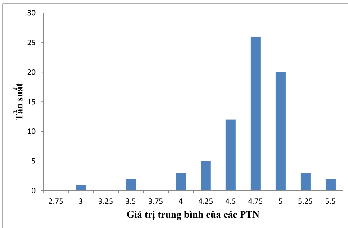
Hình 1. Biểu đồ Histogram của mẫu A
