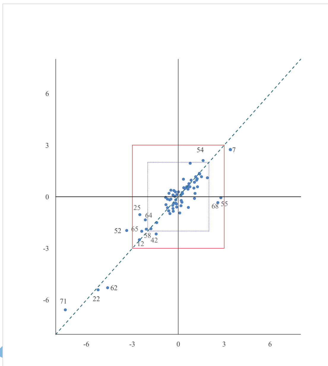
Hình 7. Biểu đồ Youden Plot của mẫu A và mẫu B
