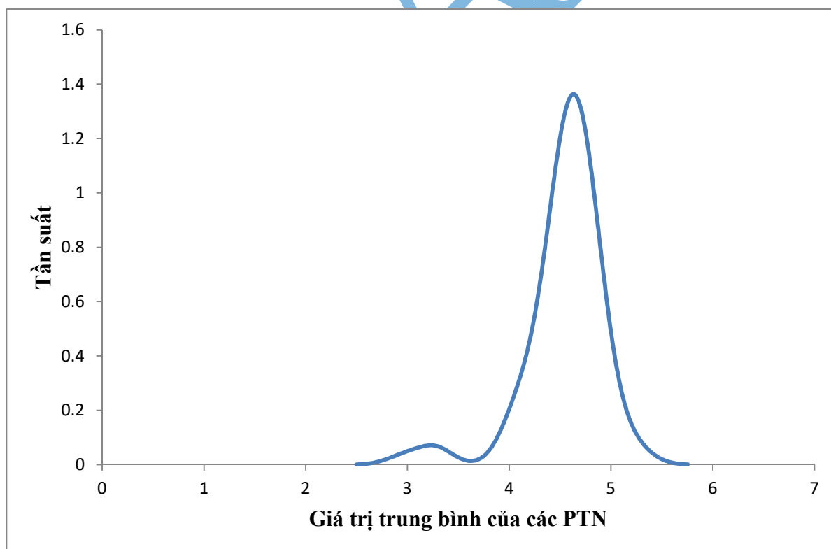
Hình 4. Biểu đồ Kernel của mẫu B
