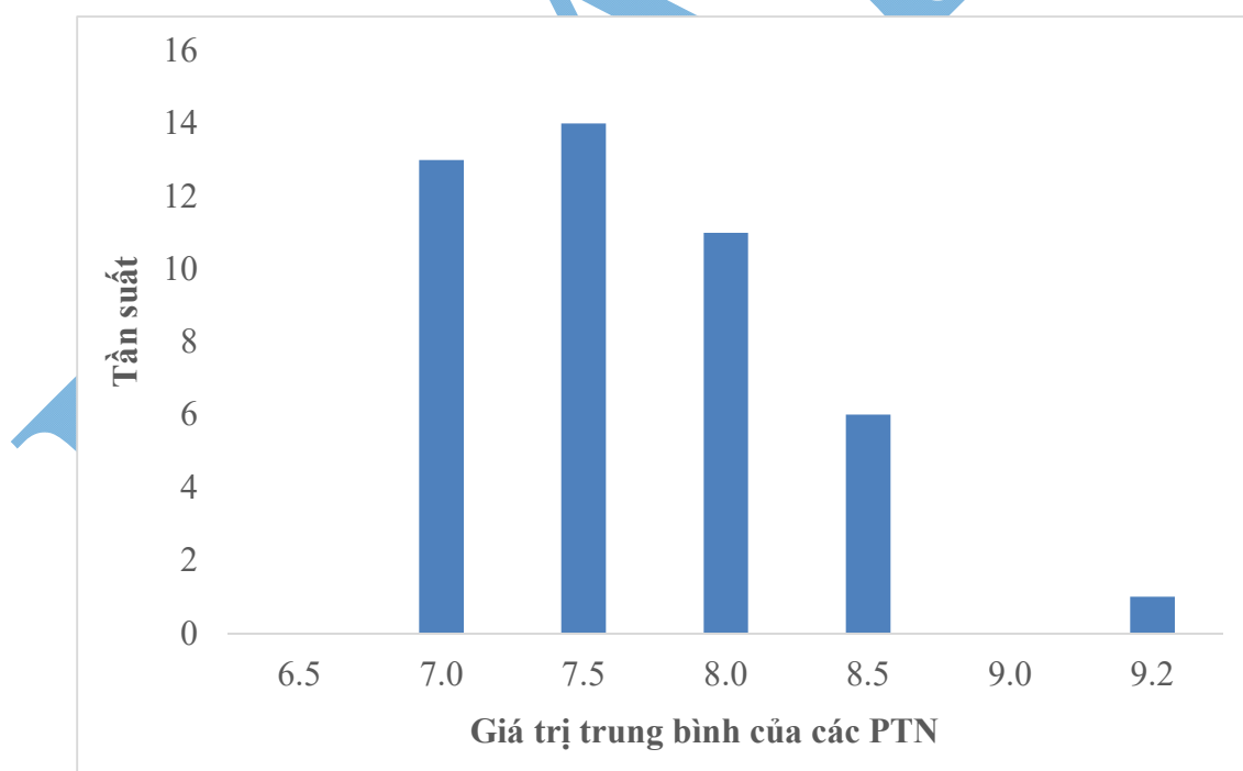
Hình 2. Biểu đồ Histogram của mẫu B
