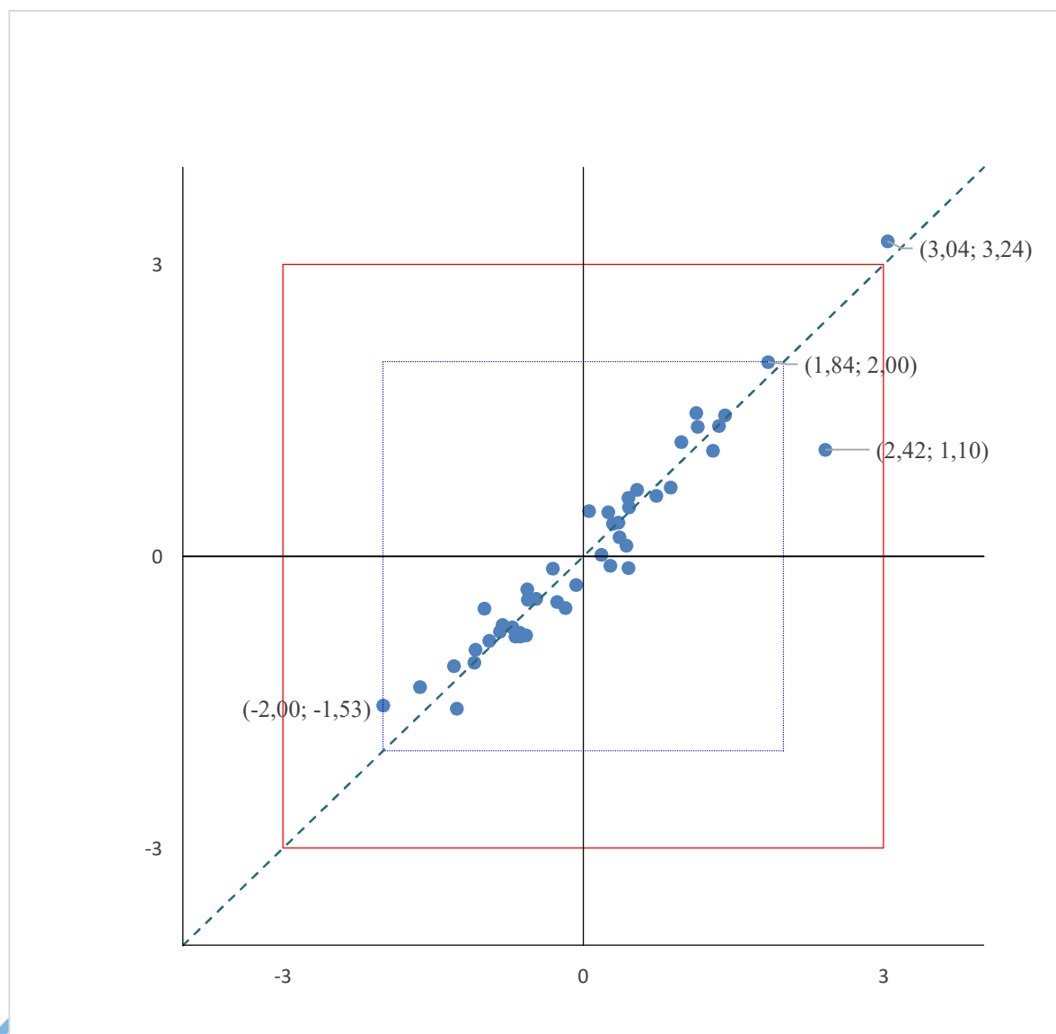
Hình 5. Biểu đồ Youden Plot của mẫu A và mẫu B
