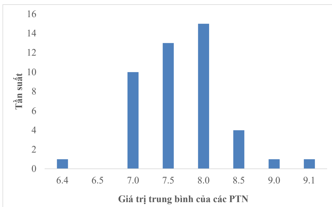
Hình 1. Biểu đồ Histogram của mẫu A
