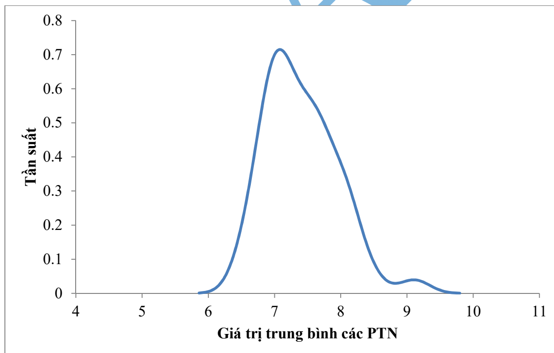
Hình 7. Biểu đồ Kernel Density Estimation của mẫu B
