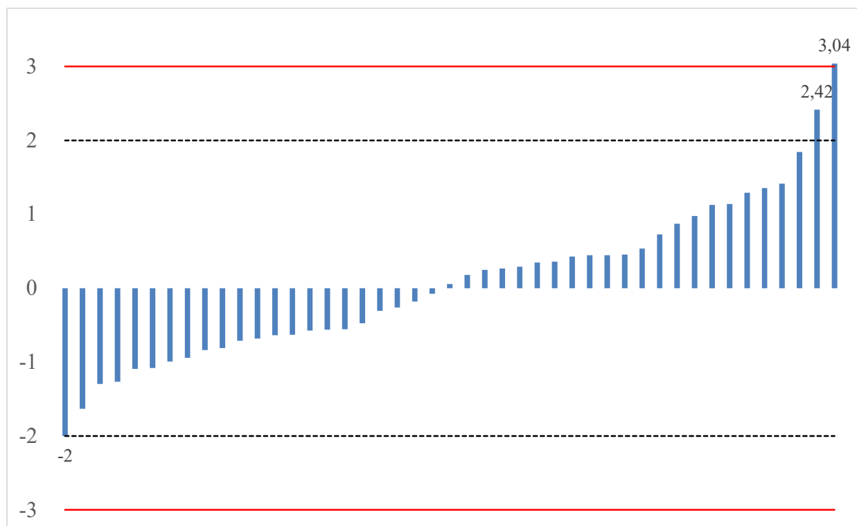
Hình 3. Biểu đồ Bar-plots của mẫu A
