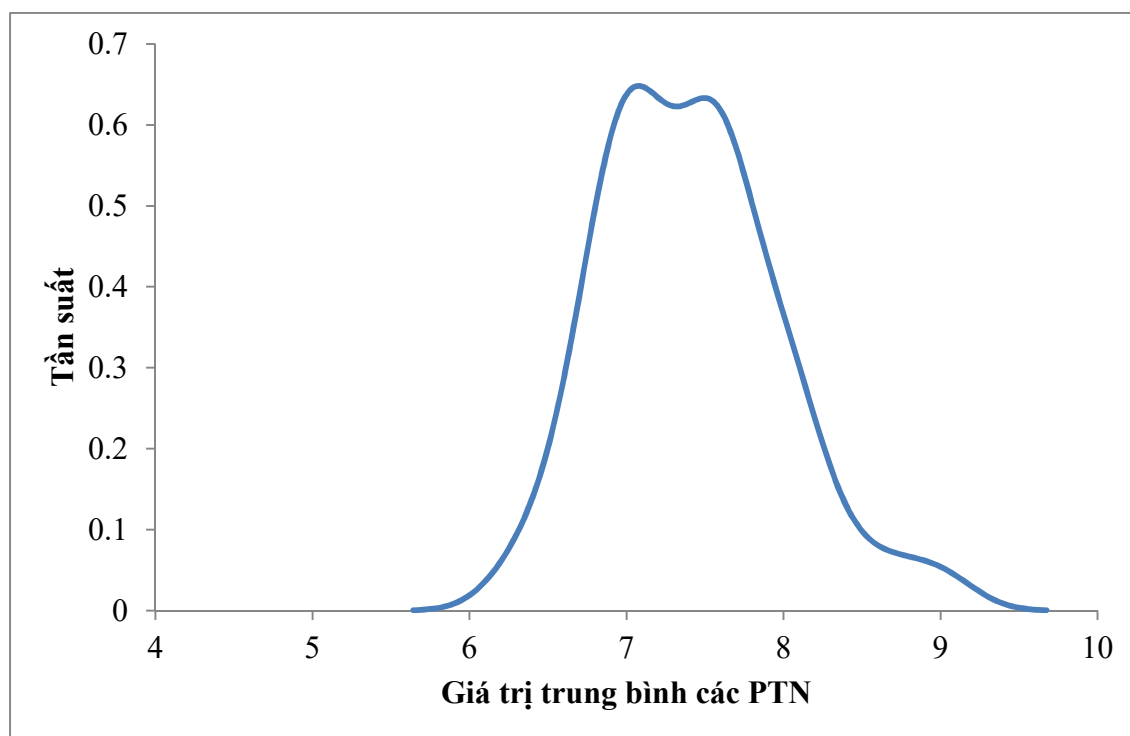
Hình 6. Biểu đồ Kernel Density Estimation của mẫu A
