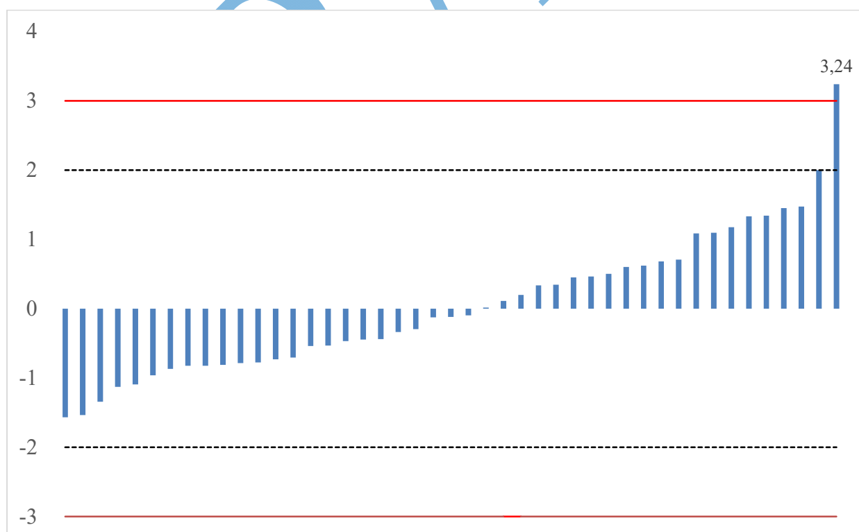
Hình 4. Biểu đồ Bar-plots của mẫu B
